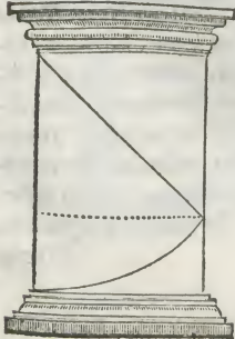
Doricus Stylobata.
